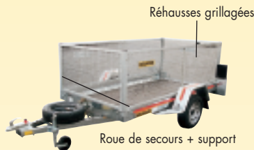
Jeu de 3 ridelles (hauteur + 400 mm)
